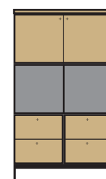
STCC31 W 760 D 380 H 1261
