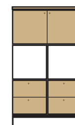
STCC32 W 760 D 380 H 1261
